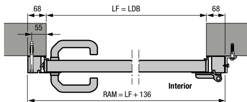
Ușă alăturată cu toc bloc de aluminiu, tip profil 1 Montaj în spatele deschiderii
