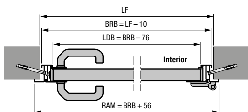
Ușă alăturată cu toc de colț de aluminiu, tip profil 1 sau 2 Opritor interior
