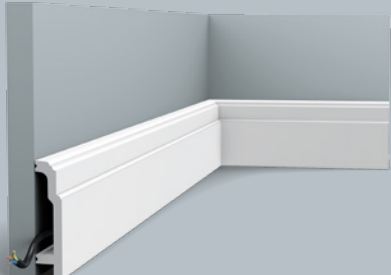
SX155 | SX155F 200 x 10,8 x 2,5 cm Duropolymer ®
