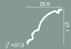
C336 BA'ROCK 200 x 27,1 x 26,6 cm Purotouch ®
