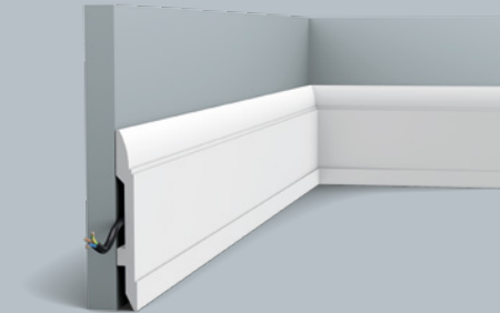
SX104 | SX104F 200 x 14,8 x 1,7 cm Duropolymer ®
