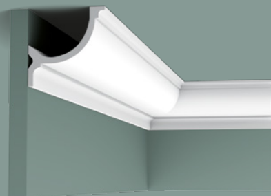
C902 | C902F 200 x 10,3 x 10,3 cm Purotouch ® 10,3 14,2
