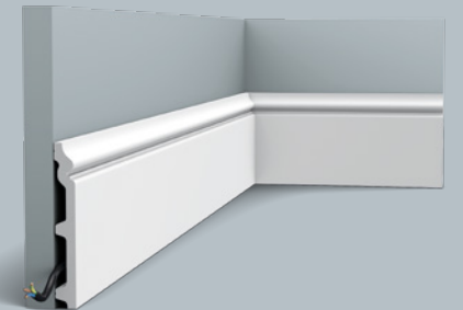
SX118 | SX118F | SX118-RAL9003 CONTOUR 200 x 13,9 x 1,8 cm Duropolymer ®
