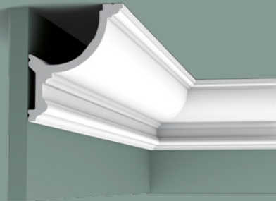
3 C901 | C901F 200 x 14,8 x 12,4 cm Purotouch ® 12,4 14,8 19,2
