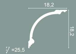
2 C338 BA'ROCK 200 x 18,2 x 18,2 cm Purotouch ®
