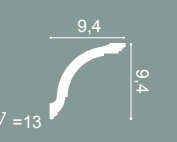
CX128 200 x 9,4 x 9,4 cm Duropolymer ®
