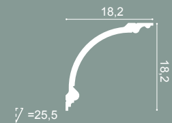
3 C338B BA'ROCK 200 x 18,2 x 18,2 cm Dessin: 2 x 57 cm Purotouch ®
