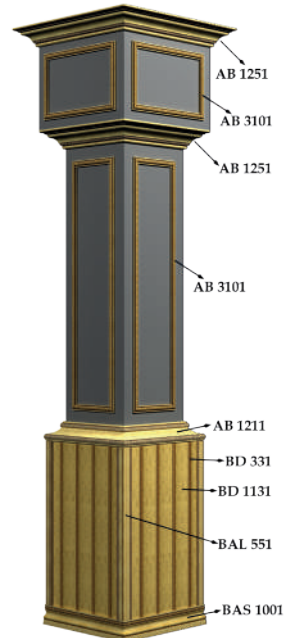
LAMBİRİ ARA PROFİLİ BD 331
