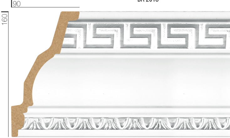
AHŞAPPIYER PROFİLİ BA 2018
