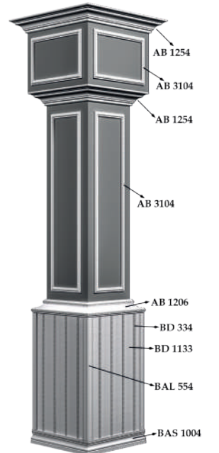
LAMBİRİ ARA PROFİLİ BD 334
