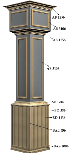
LAMBİRİ ARA PROFİLİ BD 336
